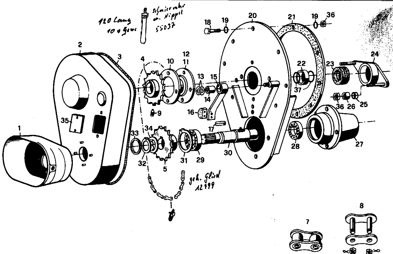
Vorgelege kpl. mit S-Sprache und Buchsen/Schinder alle Größen
